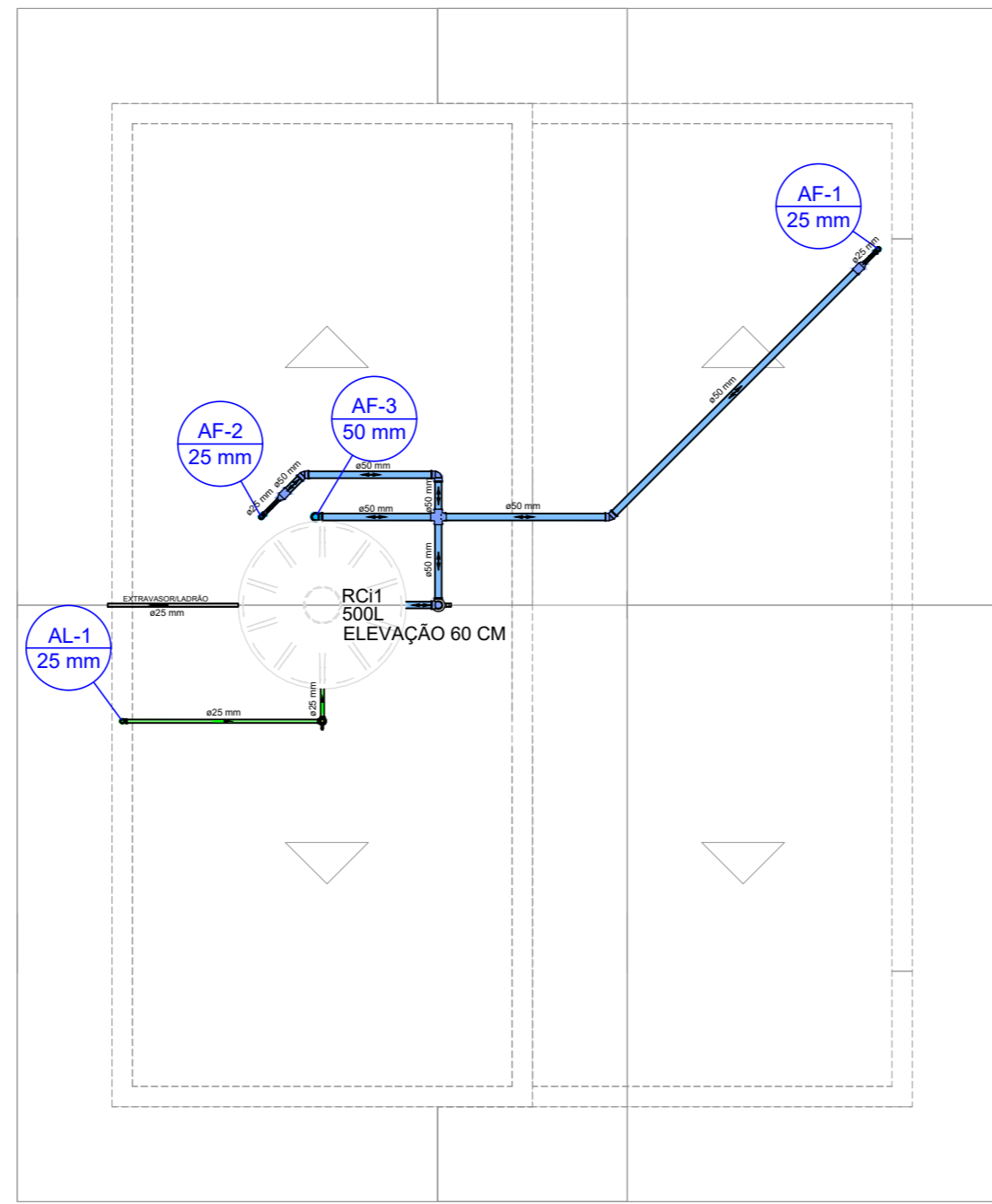
PLANTA BARRILETE 1:50
