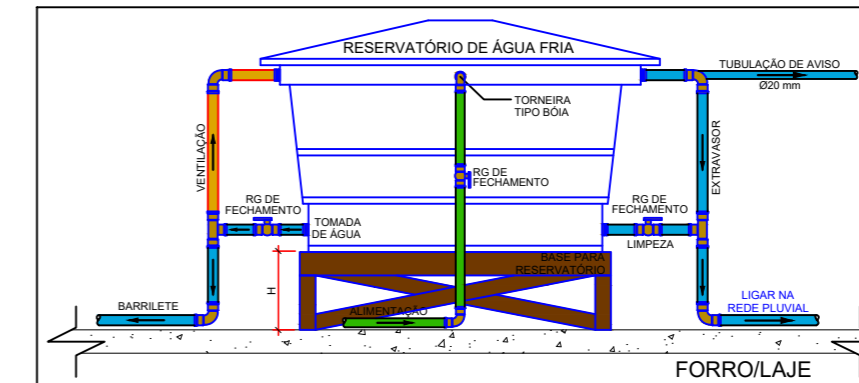
DETALHE CAIXA D'ÁGUA SEM ESCALA
