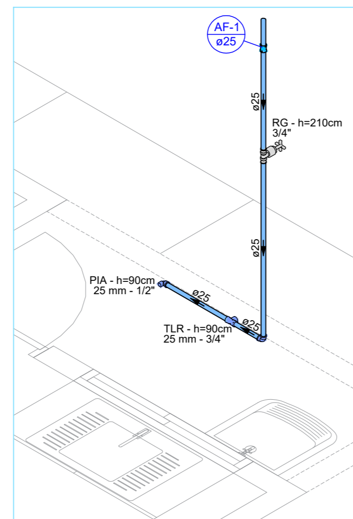
Isométrico copa e serviço 1:50
