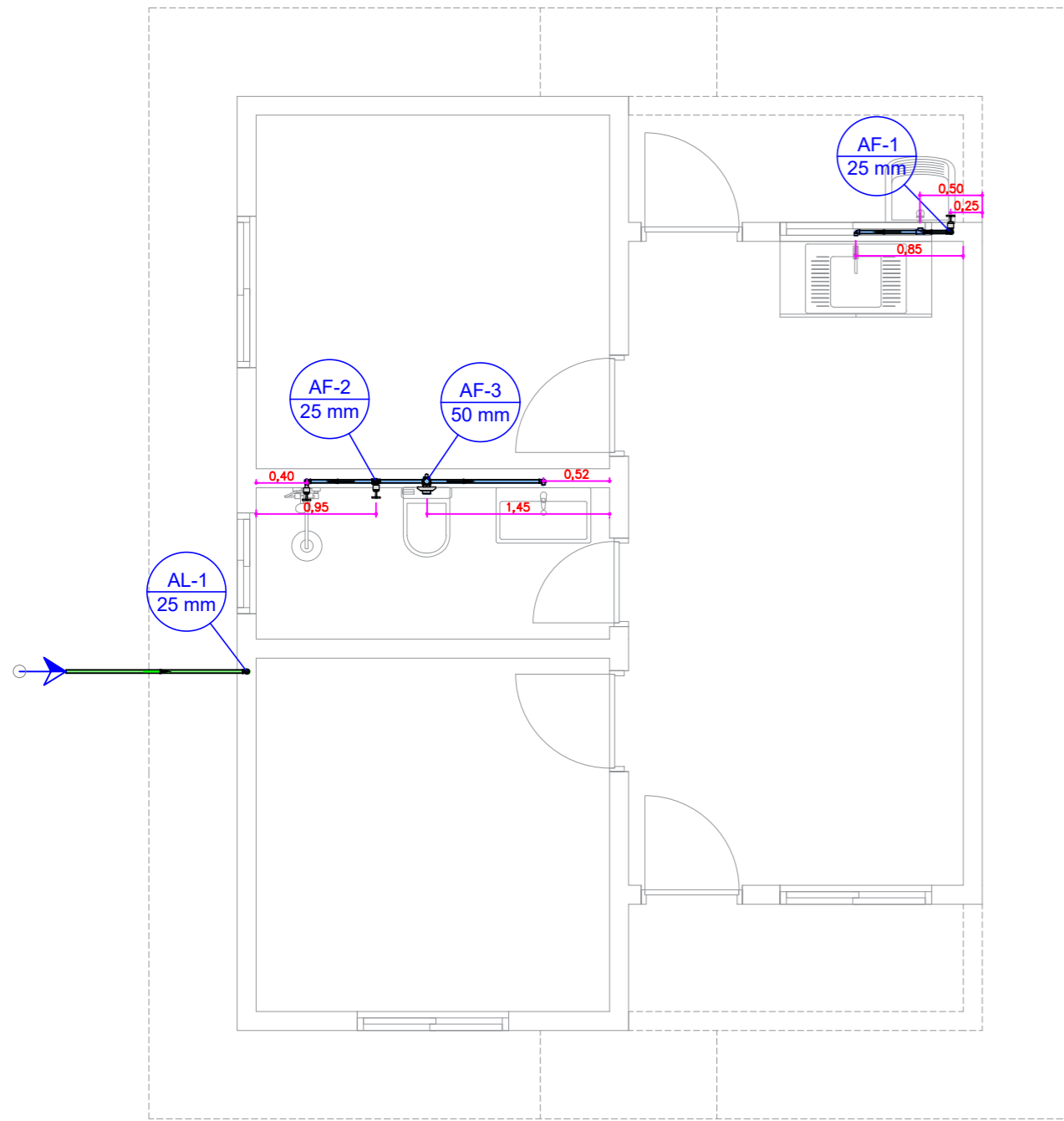
PLANTA BAIXA 1:50
