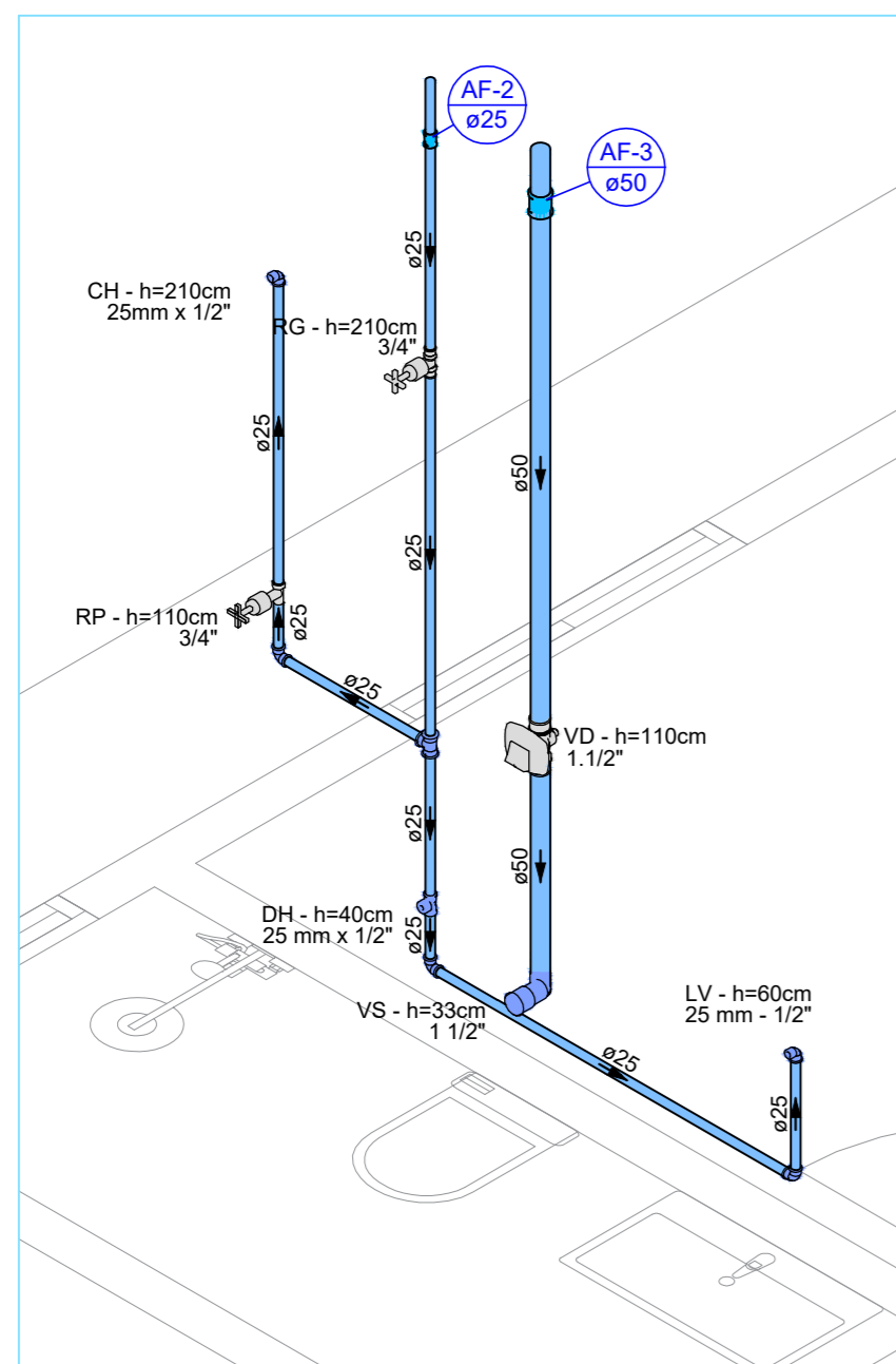
Isométrico BWC Social 1:50
